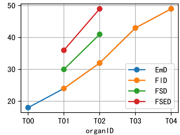
P3-6-003-24 Phe
