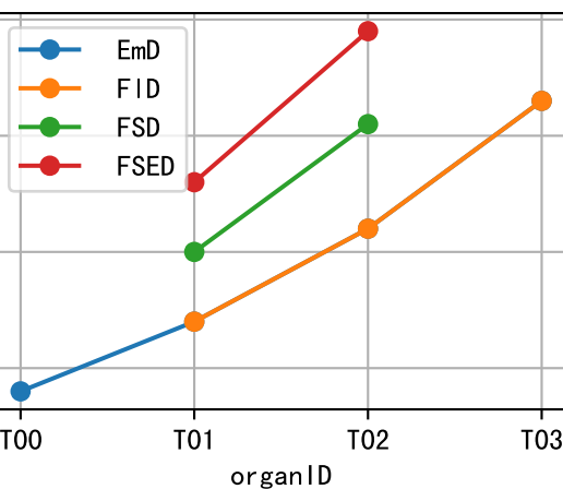
P3-6-028-32 Phe
