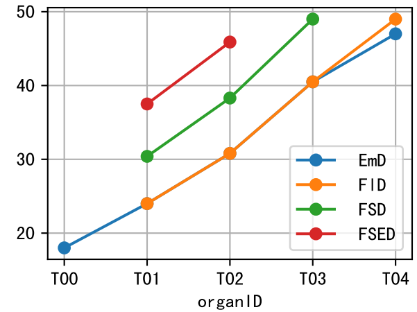
P3-6avg Phe
