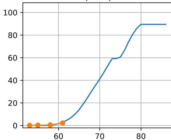
Fit(S1T4Fr5')
