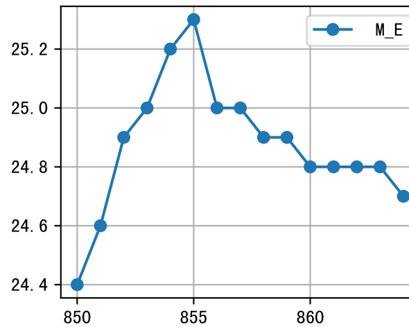
m=500, m FV0=0
