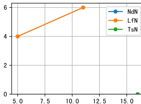
P3-045-17
