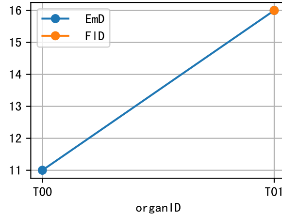
P3-110-23 Phe
