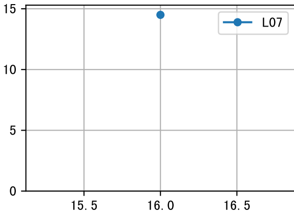
LfL (P3-009-13)
