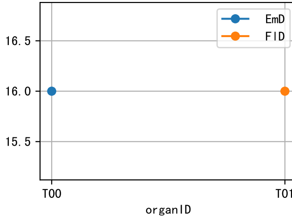
P3-099-4 Phe
