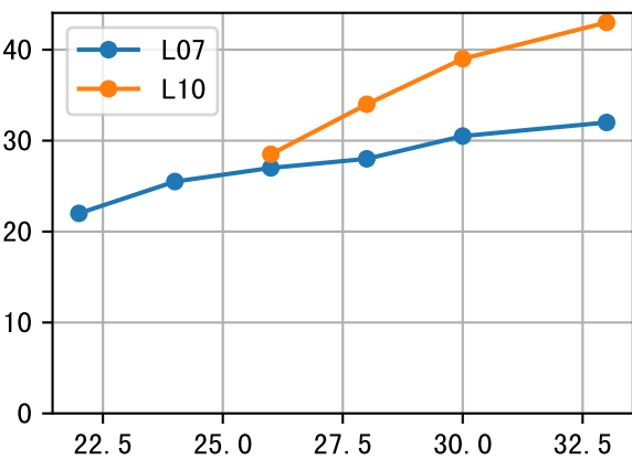
LFW (P3-054-28)
