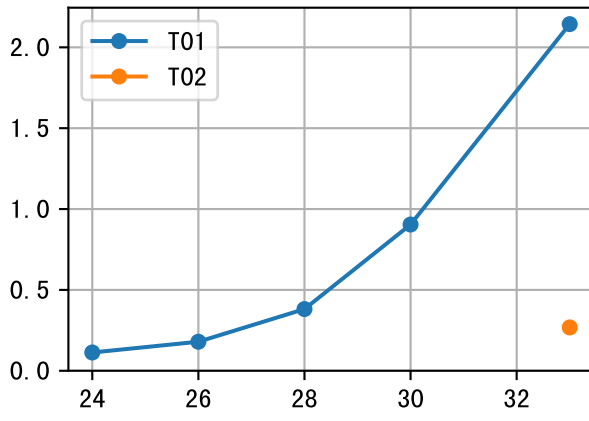
FrV (P3-054-28)
