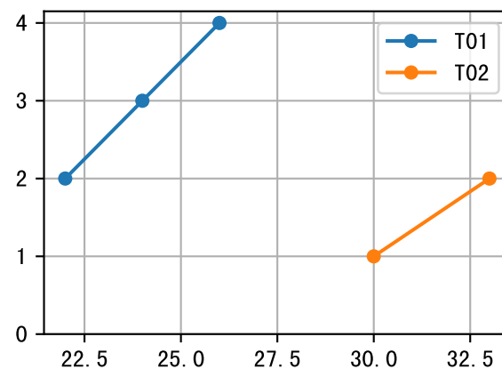
FrNR (P3-034-5)
