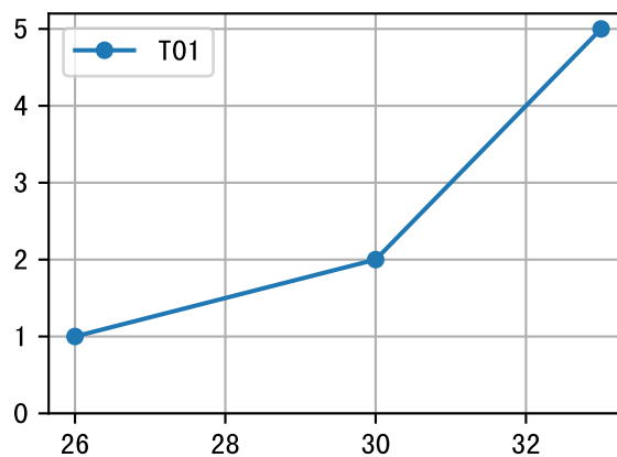
FrNR (P3-045-17)
