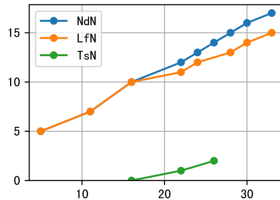
P3-054-28
