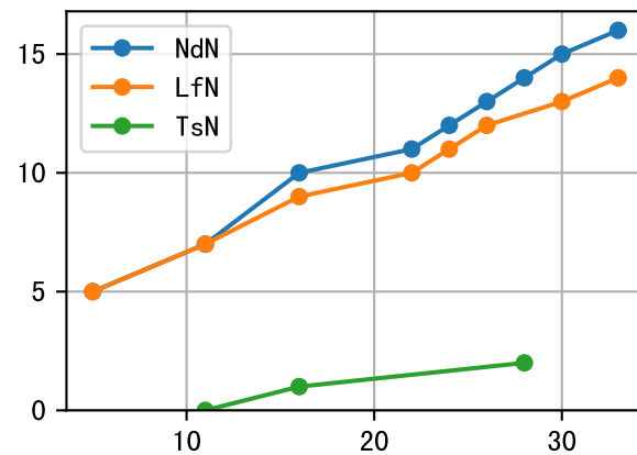
P3-084-11
