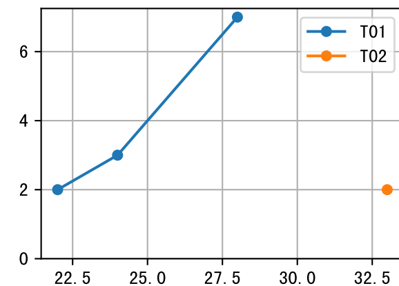
FrN (P3-009-13)
