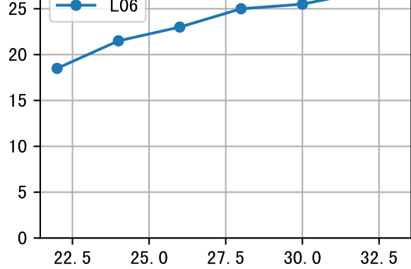
LFW (P3-045-17)
