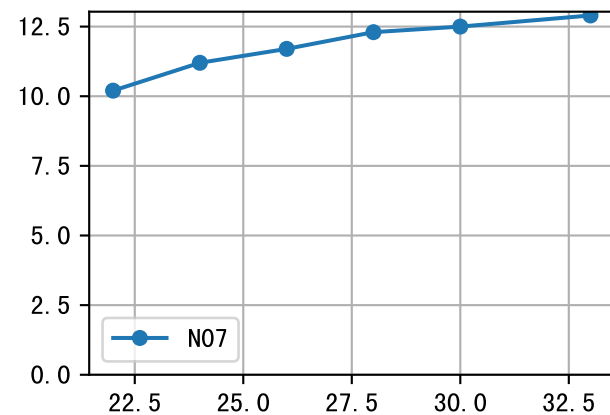
NdD (P3-045-17)
