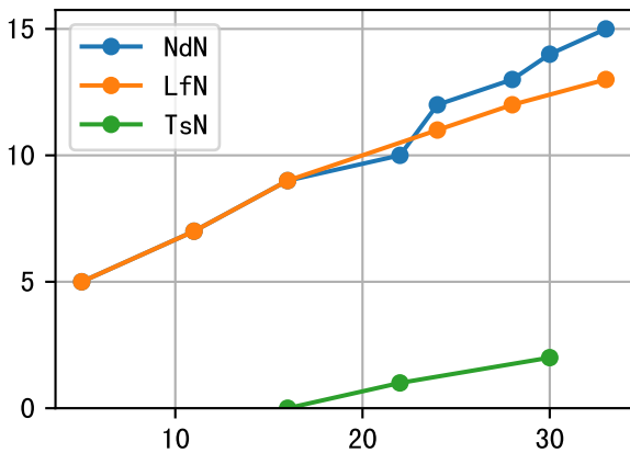
P3-099-4
