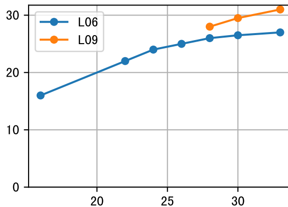
LfL (P3-084-11)
