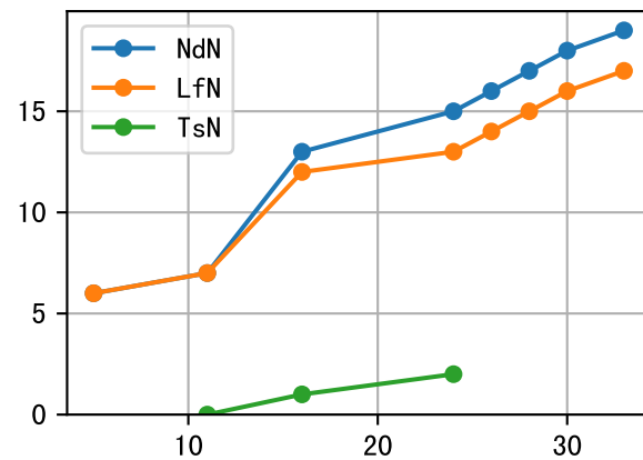
P3-021-19
