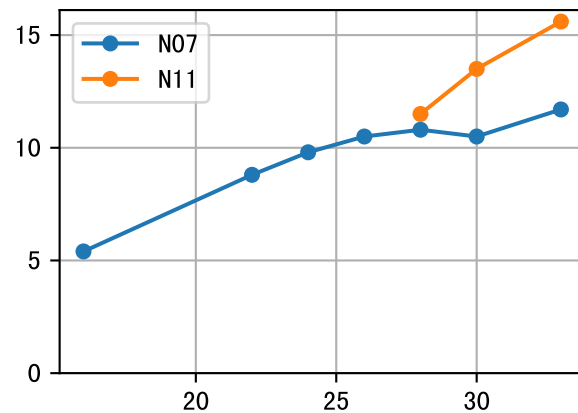
NdD (P3-084-11)
