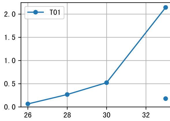
FrV (P3-045-17)
