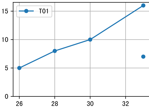
FrD (P3-045-17)
