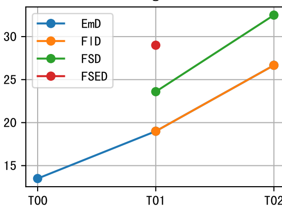
P3avg Phe
