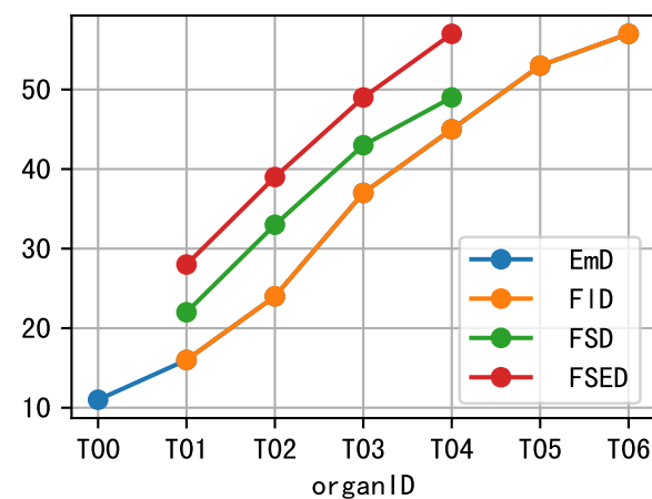
P3-021-19 Phe
