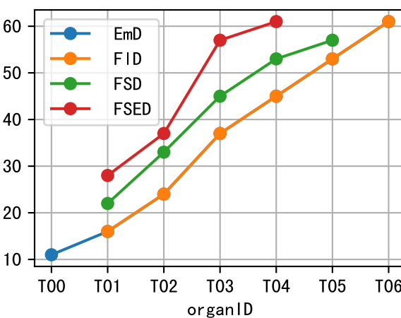
P3-009-13 Phe
