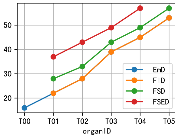
P3-075-19 Phe
