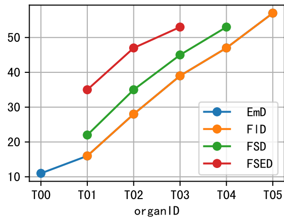
P3-084-11 Phe
