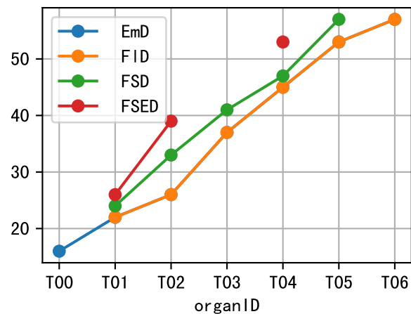
P3-054-28 Phe
