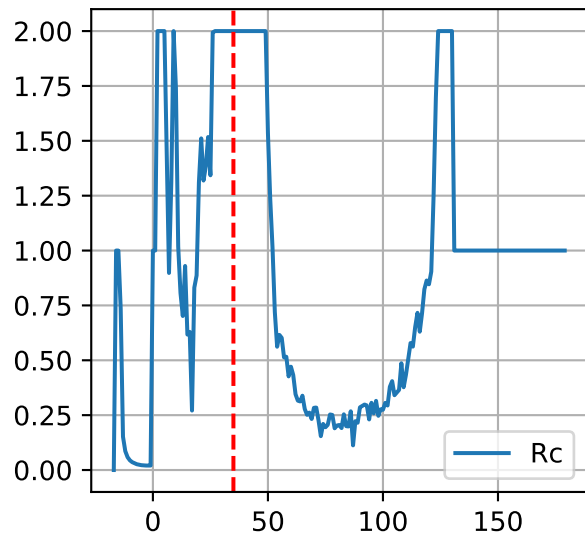
P4: ['Rc']
