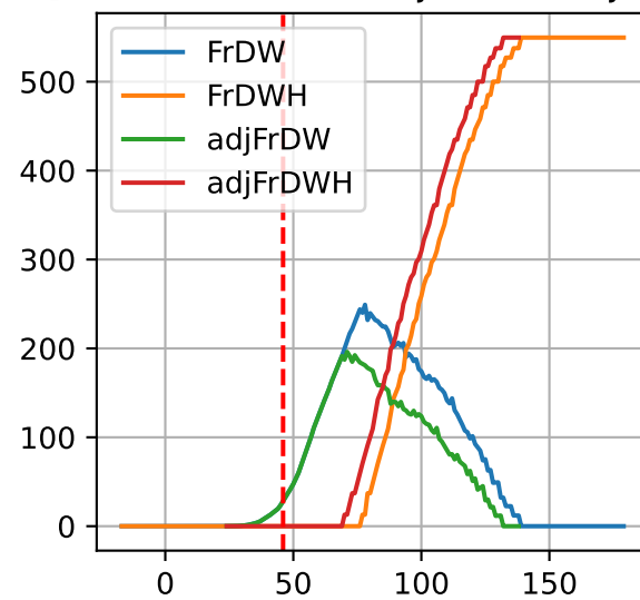
P5: ['FrDW', 'FrDWH', 'adjFrDW', 'adjFrDWH']
