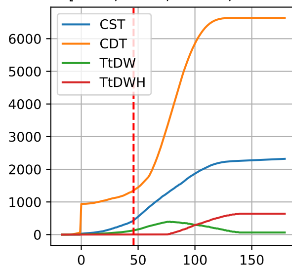
P5: ['CST', 'CDT', 'TtDW', 'TtDWH']
