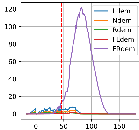
P5: ['Ldem', 'Ndem', 'Rdem', 'FLdem', 'FRdem']
