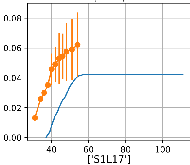
LfA (P6AE) ['S1L14']
