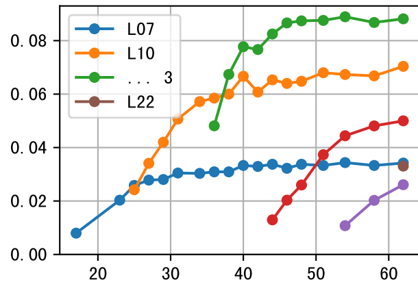
LfA (P6AE-026-25)
