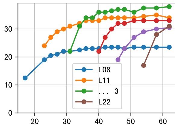
LfL (P6AE-014-17)
