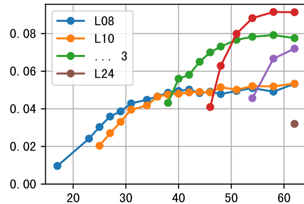
LfA (P6AE-033-4)
