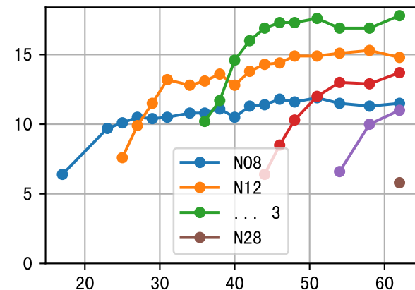
NdD (P6AE-026-25)
