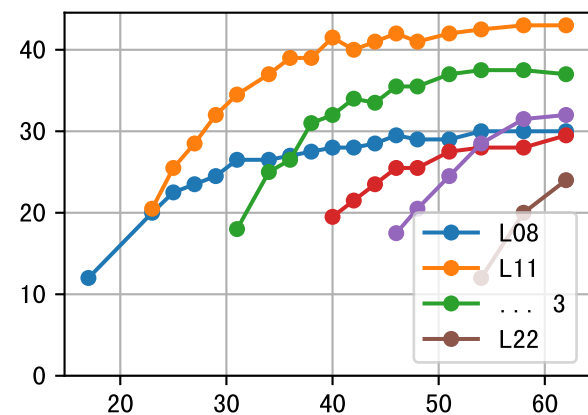
LfW (P6AE-014-17)
