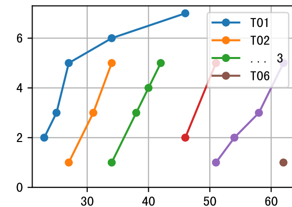
FrN (P6AE-014-17)
