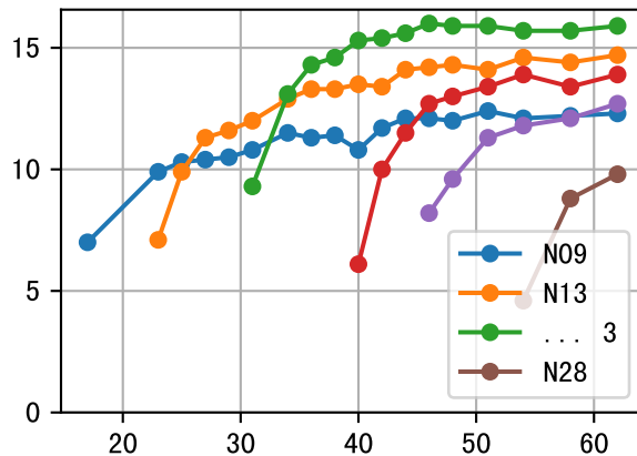
NdD (P6AE-014-17)
