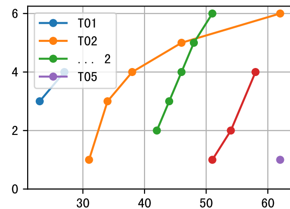
FrN (P6AE-026-25)
