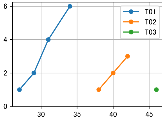
FrN (P6AW-087-14)
