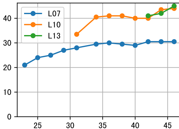
LfL (P6AW-087-14)
