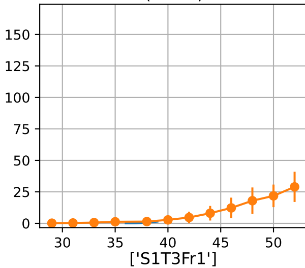
FrVSp1Fr5
