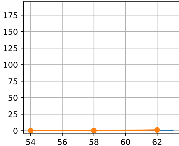
FrV(S1T4Fr5)
