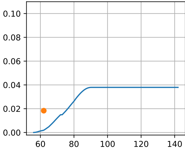
LfA['S1L20']
