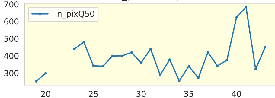
n_pixQ50 day
