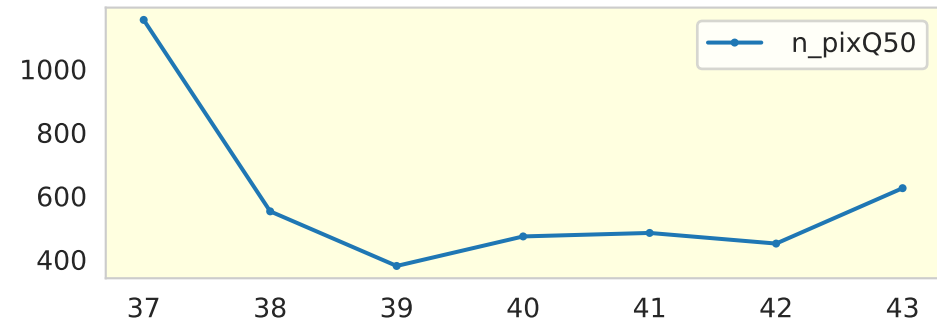
n_pixQ50 day
