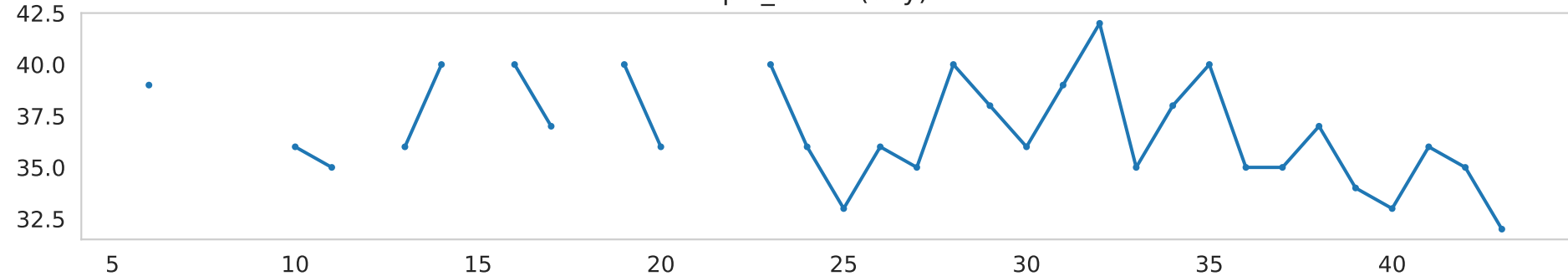
pic_count (day)
