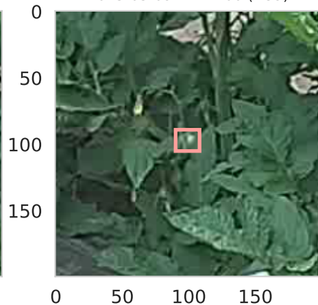
2025-05-13 15:54:00 (D43)
