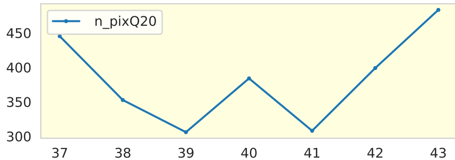
n_pixQ20 day
