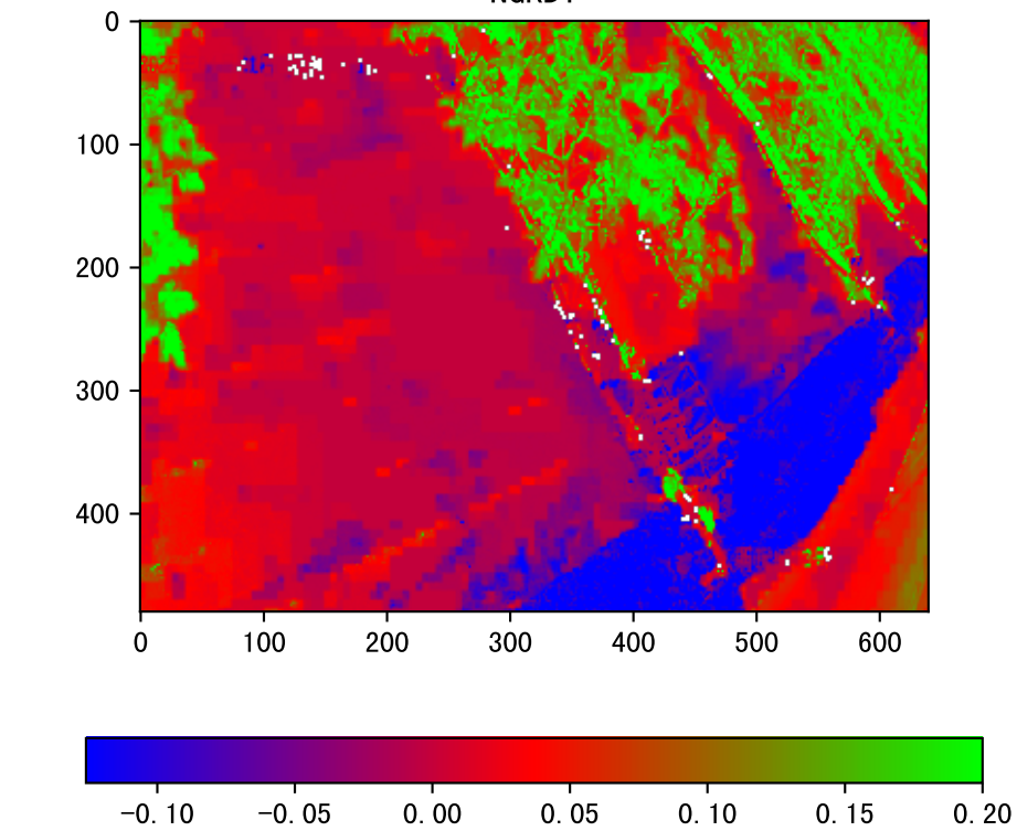
NGRDI
