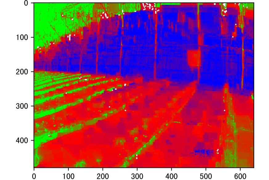
NGRDI
