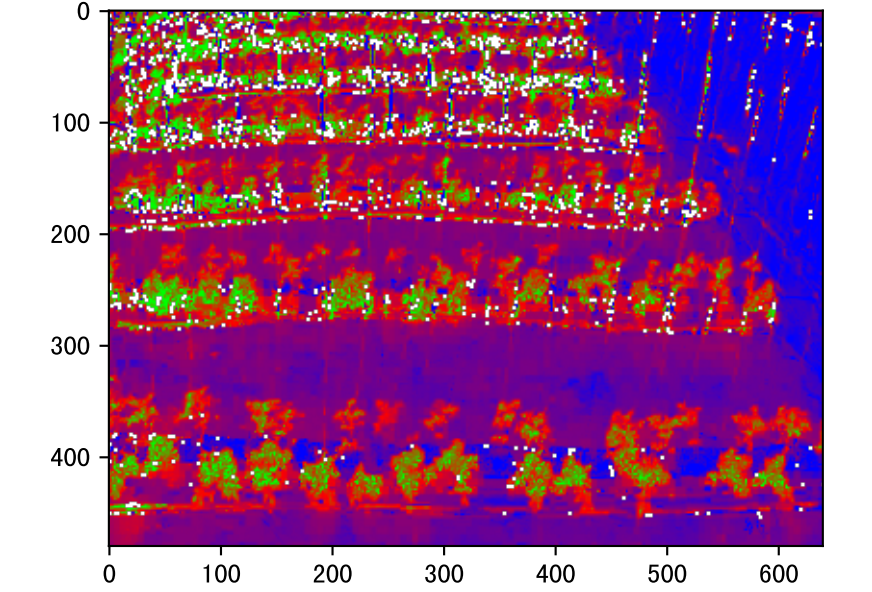
VARI
