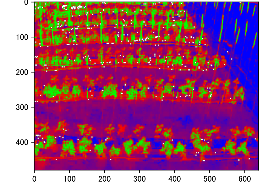
NGRDI
