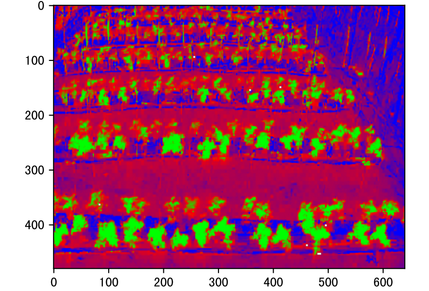
GLI
