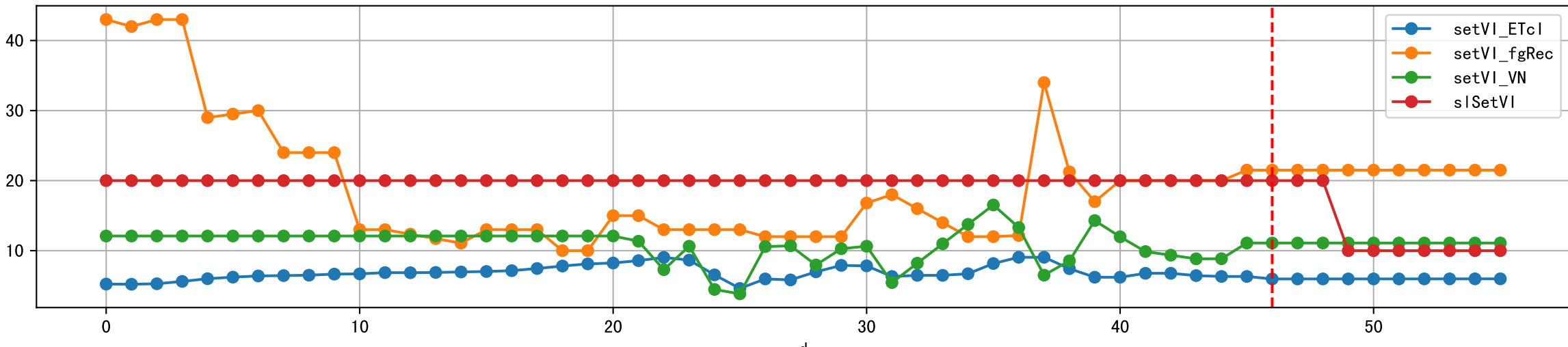
Plot [['setVI_ETcI', 'setVI_fgRec', 'setVI_VN', 'sISetVI']]
