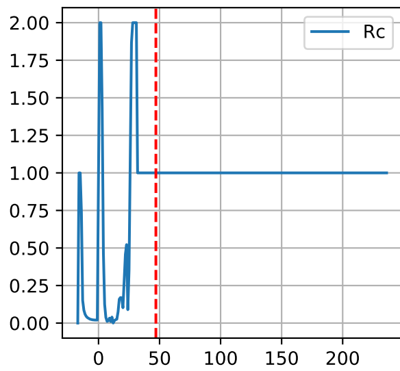
L1A3: ['Rc']
