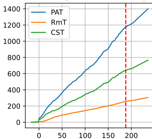
L1AC3: ['PAT', 'RmT', 'CST']
