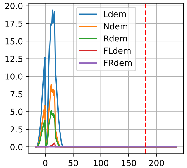
L1AC4: ['Ldem', 'Ndem', 'Rdem', 'FLdem', 'FRdem']
