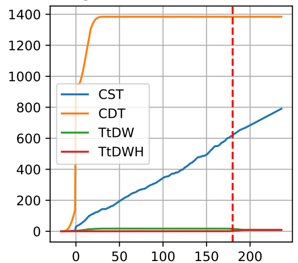
L1AC4: ['CST', 'CDT', 'TtDW', 'TtDWH']
