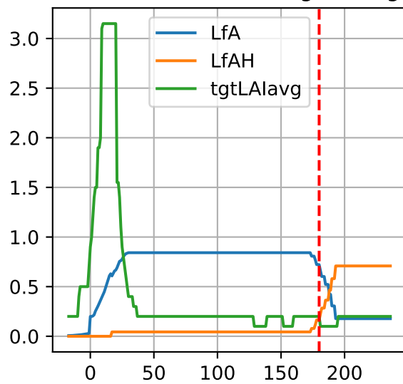
L1AC4: ['LfA', 'LfAH', 'tgtLAlavg']
