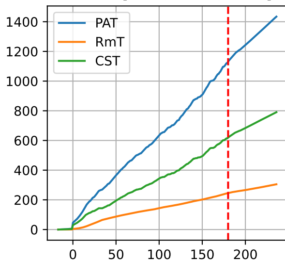
L1AC4: ['PAT', 'RmT', 'CST']
