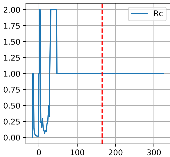
XX8: ['Rc']
