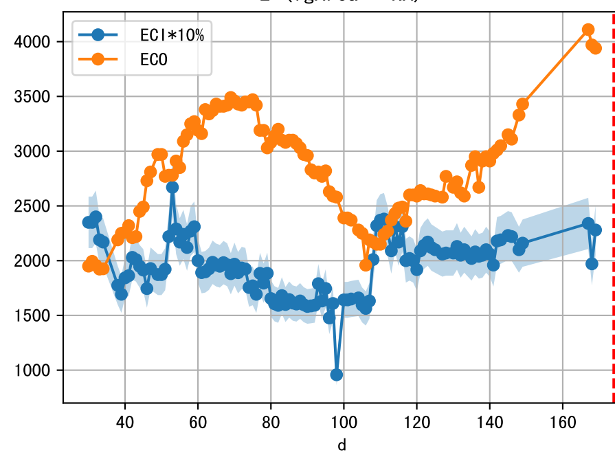
2 (fgArea = NA)
