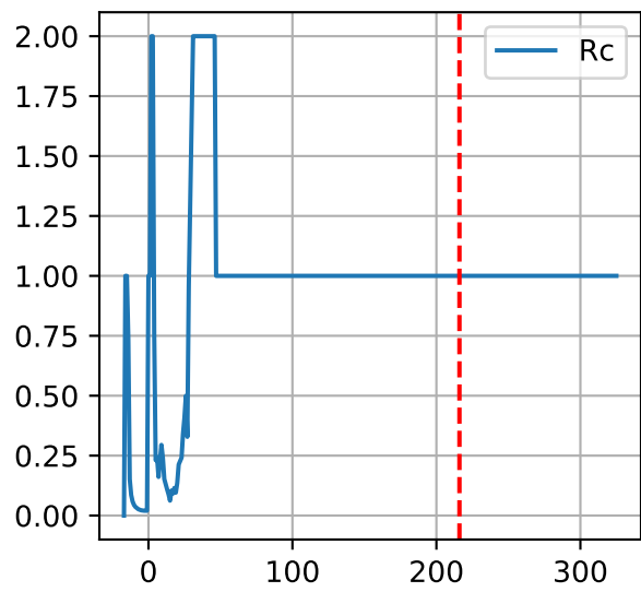
XX8: ['Rc']
